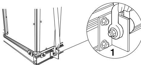
Figur: Løftepunkt forhåndsmontert på bjelkeramme
