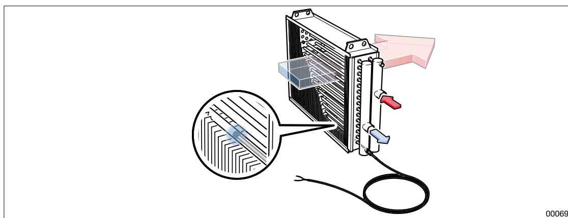
Figur: Batteri med samlerør for utgående væske, med innstikksføleren montert i drenerings-/tappenippelen.
