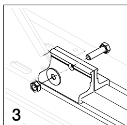
3. Spenne, (60-profil)
