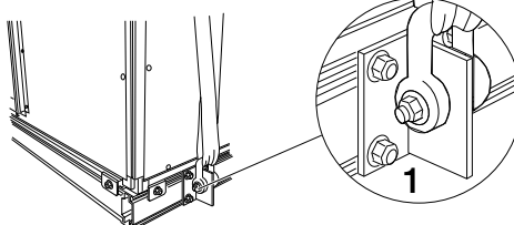
Figur: Løftepunkt forhåndsmontert på bejelkeramme
