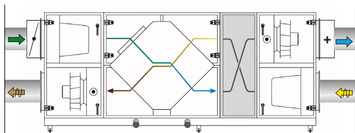
Ny installasjon, med luftvender
